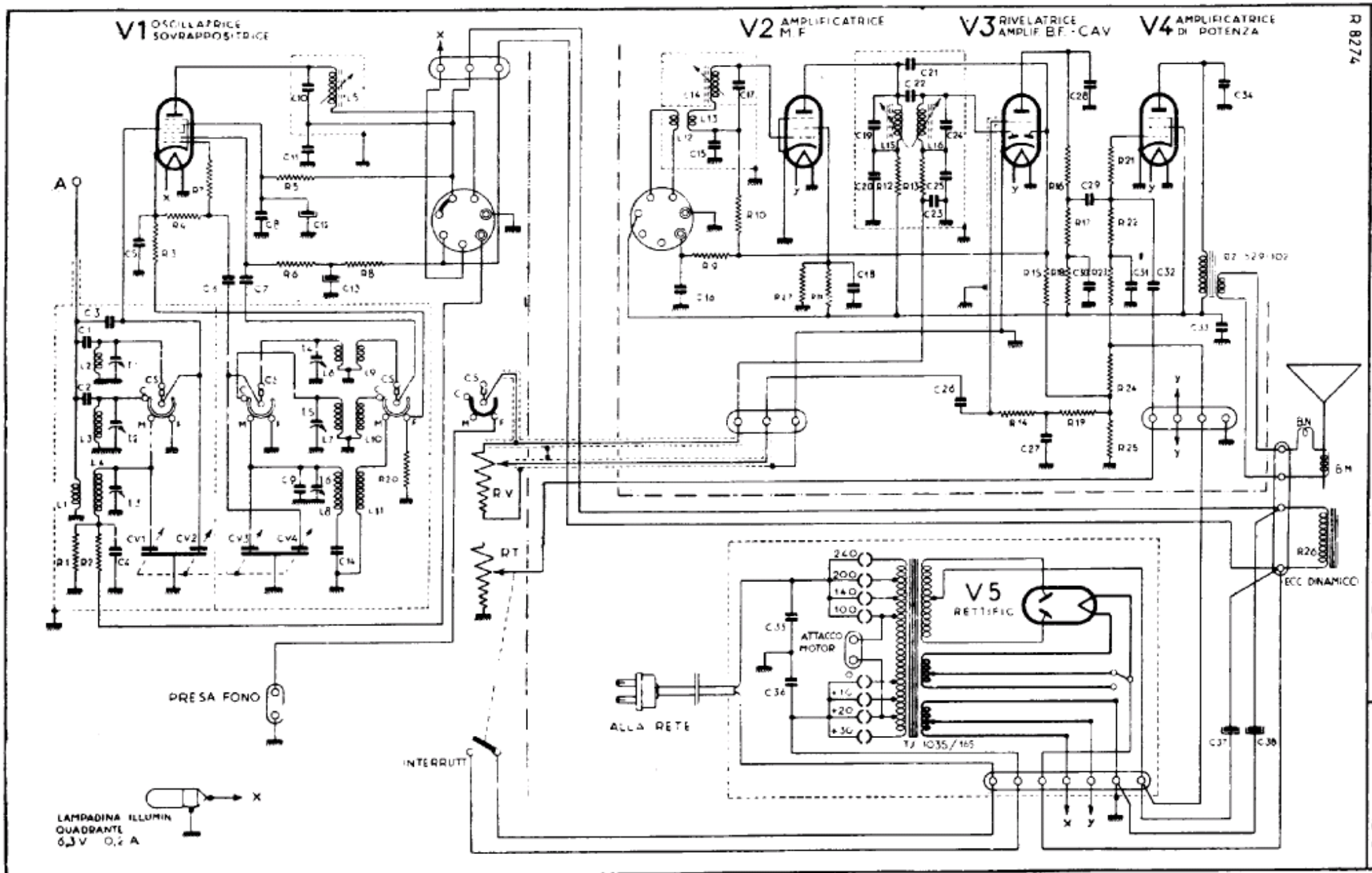
— PHONOLA (S. A. FIMI). — Mod. 523. — Serie ultraferrosite. — Produzione 1938-39. — Media frequenza: 470 kHz.
